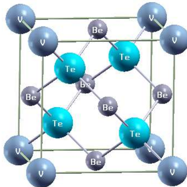
Figure IV.4: Structure cristallographique de la supercelle de 8 atomes du matériau \text{Be}_{0.75}\text{V}_{0.25}\text{Te} .
