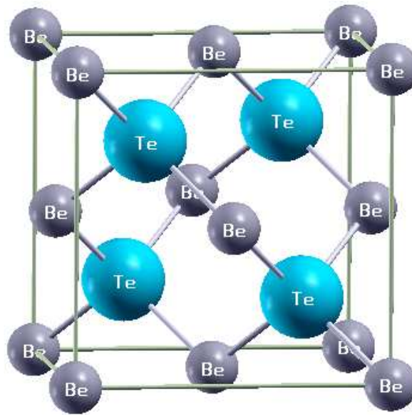
Figure IV.3 : Structure cristalline zinc blende de BeTe
