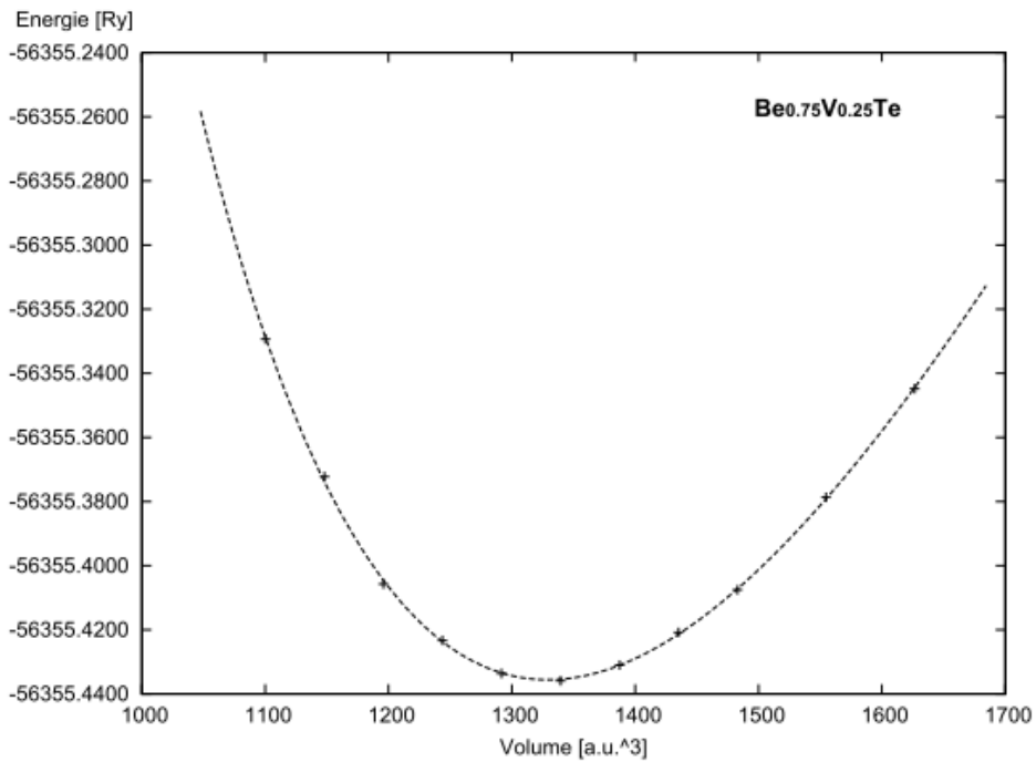
Figure IV.6 : Variation de l'énergie totale de \text{Be}_{0.75}\text{V}_{0.25}\text{Te} en fonction du volume.
