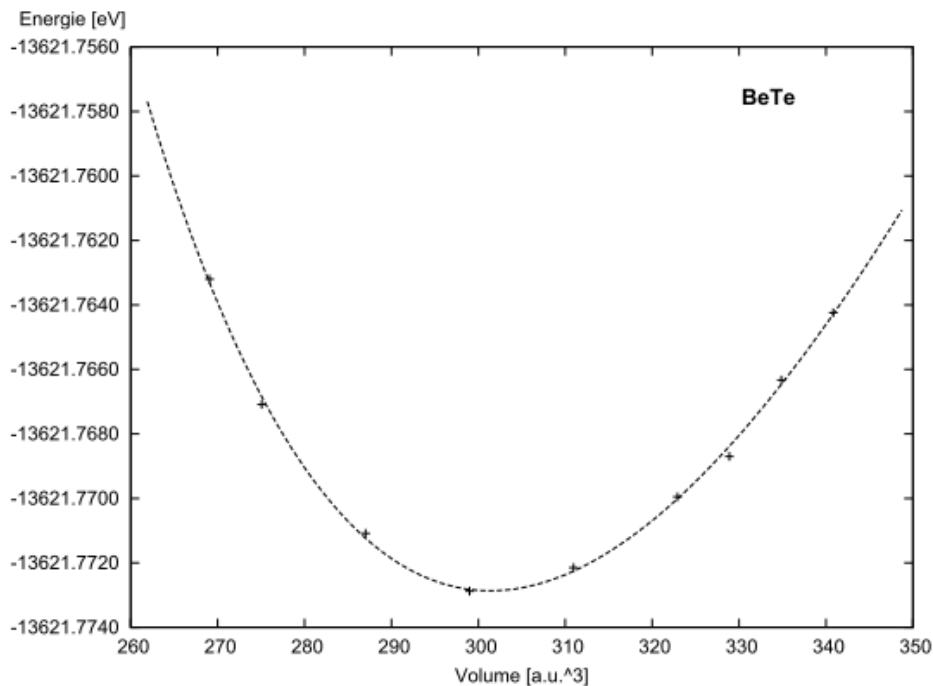
Figure IV.5 : Variation de l'énergie totale de BeTe en fonction du volume.
