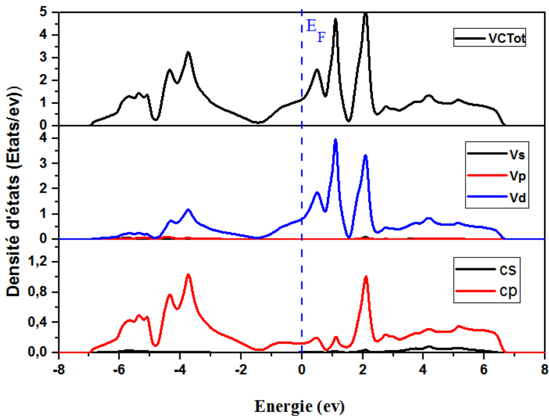
Figure III.5: la densité d'état totale (TDOS) du VC.
