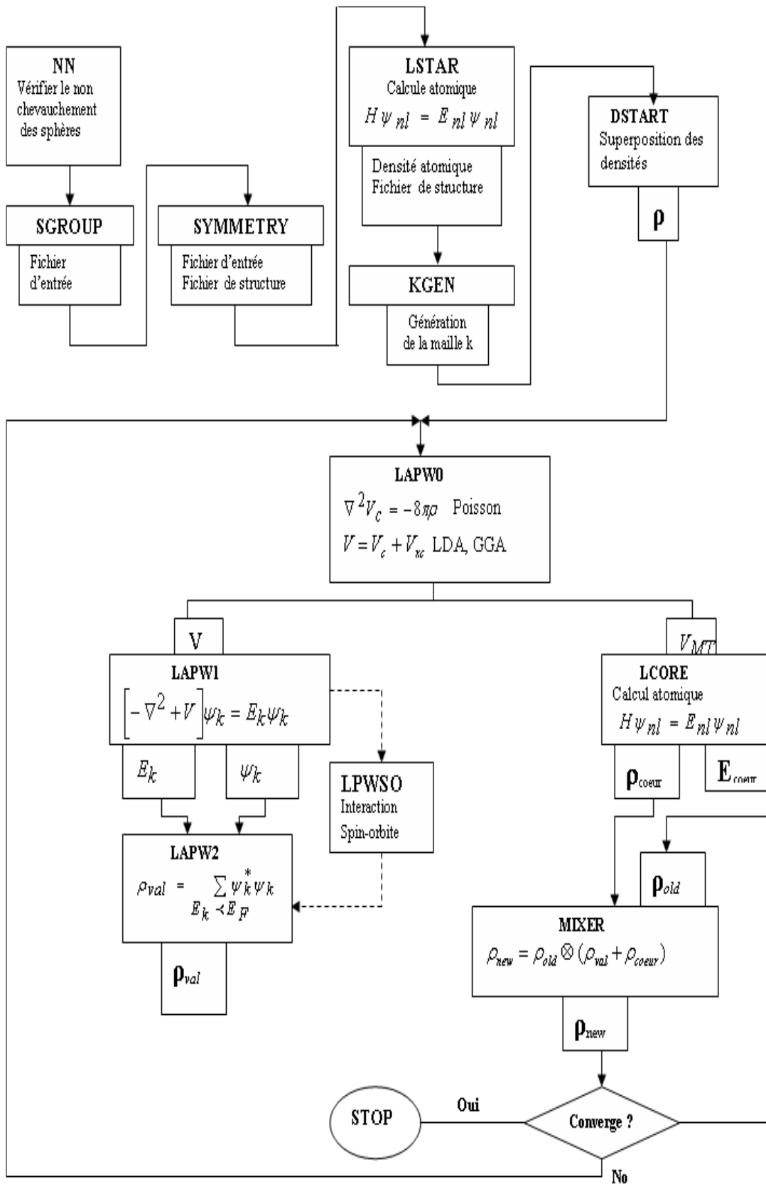
Figure II.2 : Organigramme du code WIEN2k [4].
