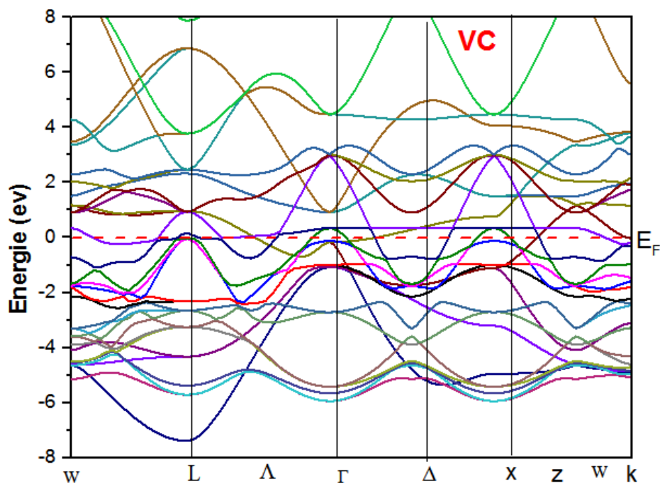
Figure III.3: La structure de bande électronique de VC.
