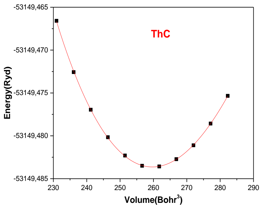
Figure III.2 : La variation de l'énergie totale en fonction du volume du ThC.
