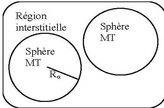
Figure II.1: Potentiel « Muffin-Tin »
