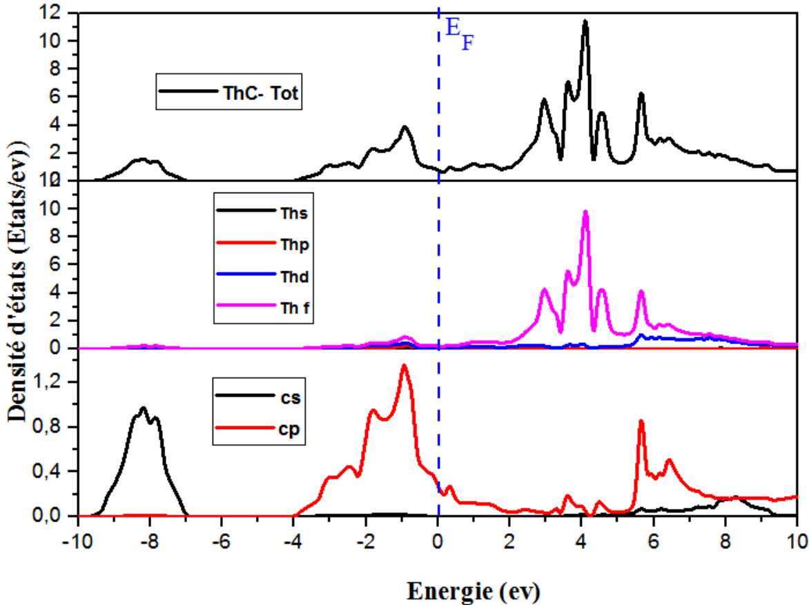
Figure III.6: la densité d'état totale (TDOS) du ThC.
