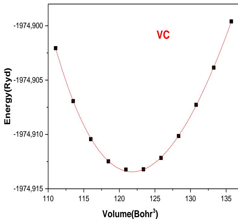
Figure III.1 : La variation de l'énergie totale en fonction du volume du VC.
