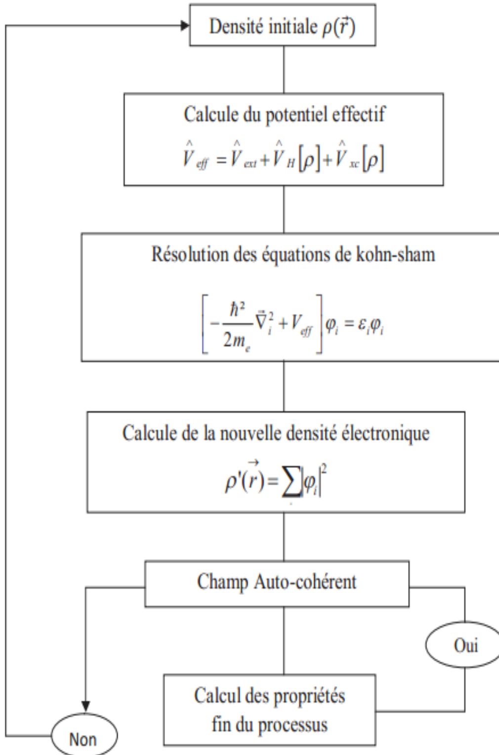
Fig I.2 : Processus auto-cohérent de kohn et sham
